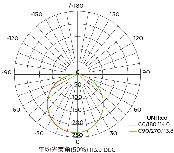
配光曲线
